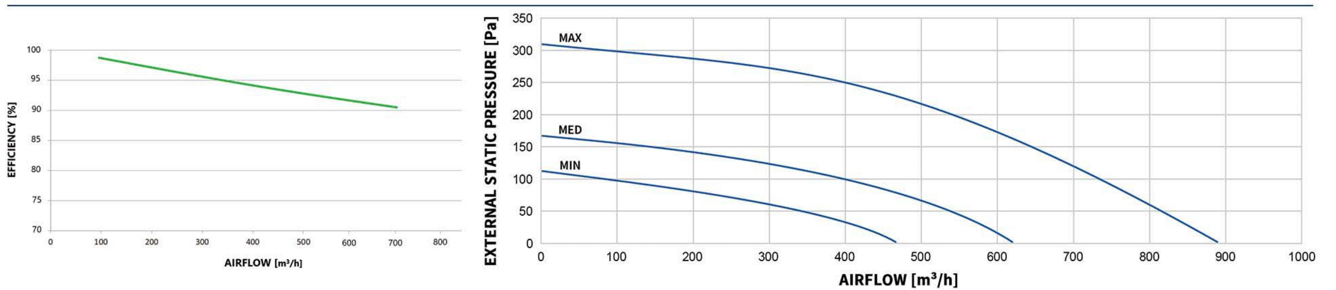
MODEL: W700-ERV-B-Z-EC
